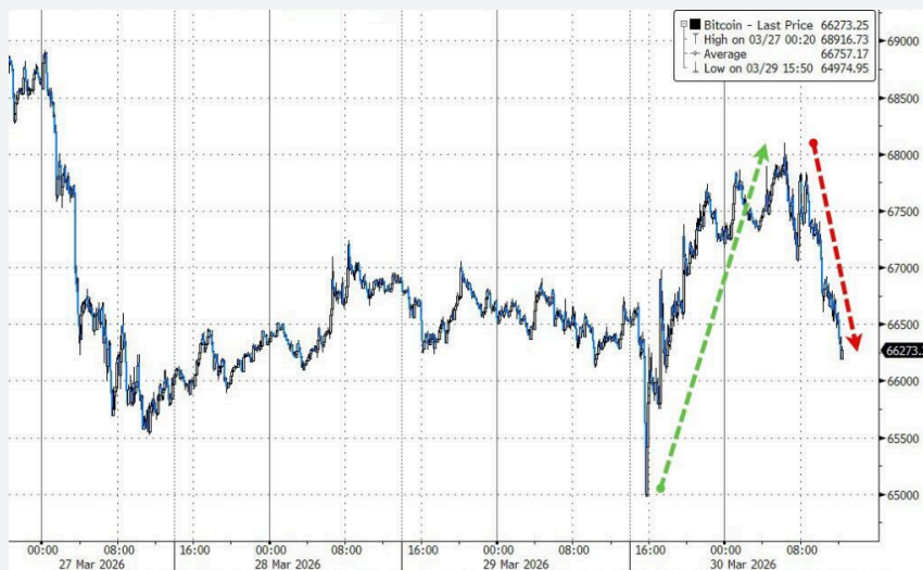
(比特币价格)
